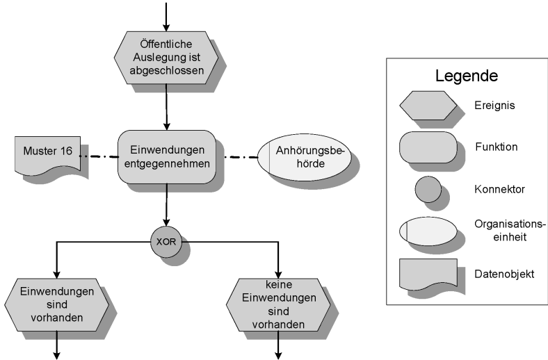
Abbildung 1: Beispiel einer erweiterten ereignisgesteuerten Prozesskette (links) und Überblick der verwendeten Knotentypen (rechts). Das alternative Eintreten der Ereignisse „Einwendungen sind vorhanden“ und „keine Einwendungen sind vorhanden“ steuert den Kontrollfluss.
