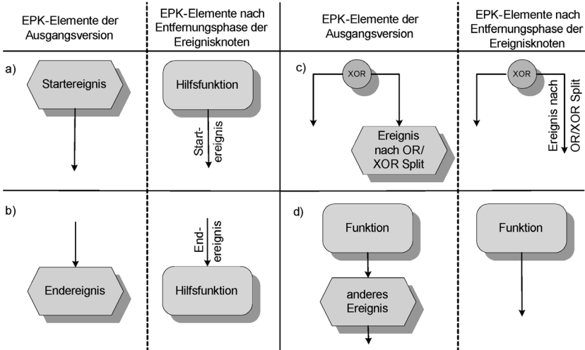
Abbildung 3: Elemente einer EPK vor und nach der Ereignisentrferungsphase für die Fälle a) Startereignis, b) Endereignis, c) Ereignis nach OR/XOR-Split und d) alle übrigen Fälle.
