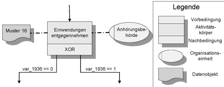
Abbildung 2: Beispiel einer transformierten Workflowbeschreibung im XPDL-Format (links) und Übersicht der verwendeten Knotentypen (rechts). Der Inhalt der Prozessvariablen var_1936 steuert den weiteren Ablauf des Workflows.
